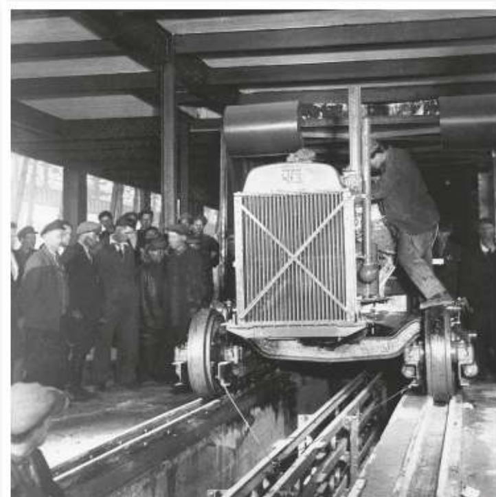
Установка карбюраторного двигателя на лигроиновом топливе на один из первых тракторов ЧТЗ. 1933 год
